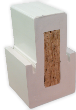
Composite T-Post
